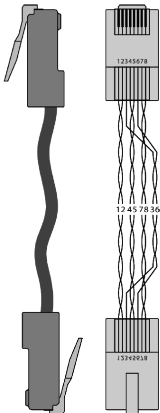
Рис. 4. Разводка CAT 5
