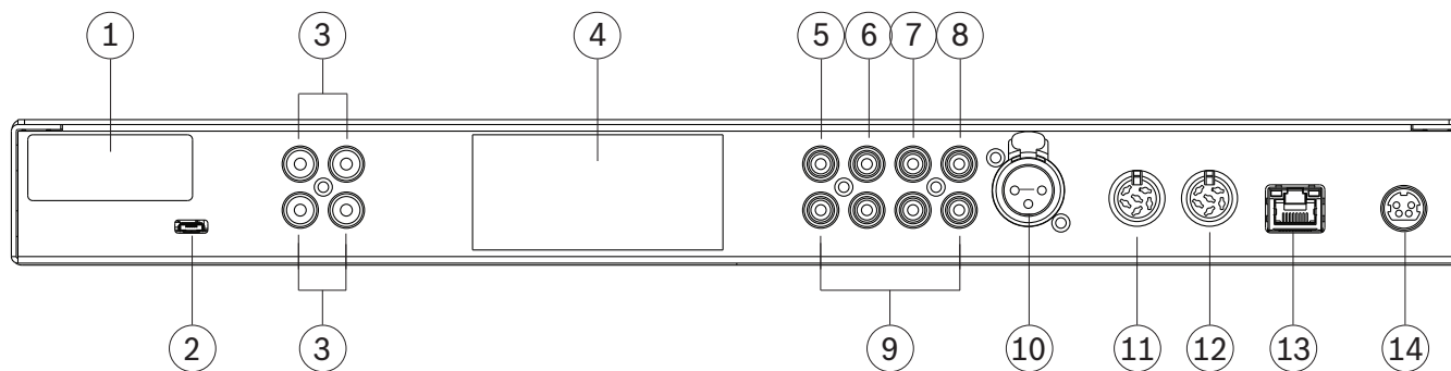
Рис. 6.2: CCSD-CURD вид сзади
