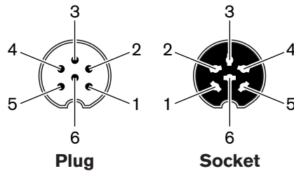
Рис. 4.2: Номера контактов на штекерном и гнездовом разъемах
