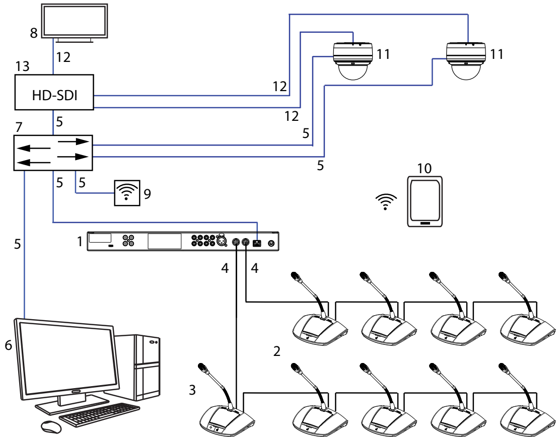
Рис. 3.1: Настройка типовой системы
