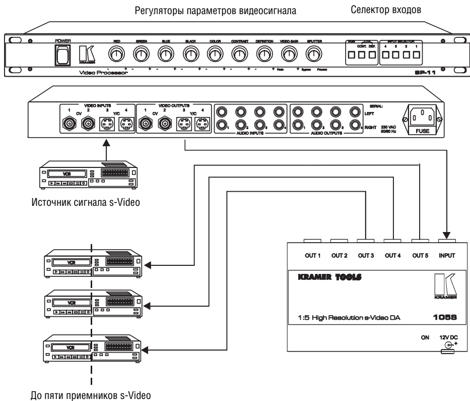
Рис. 12. Распределение видеосигнала с коррекцией параметров
