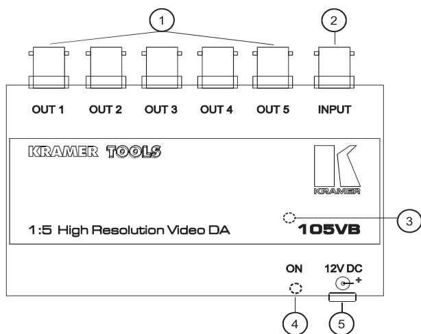
Рис. 6. Усилитель-распределитель 105VB
