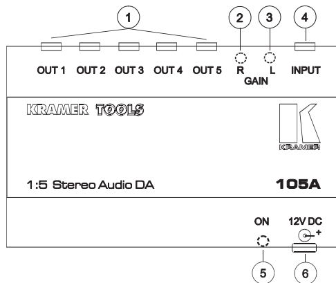
Рис. 3. Усилитель-распределитель 105A
