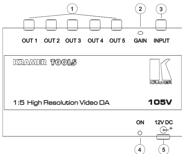
Рис. 5. Усилитель-распределитель 105V
