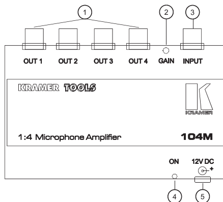
Рис. 2. Усилитель-распределитель 104M
