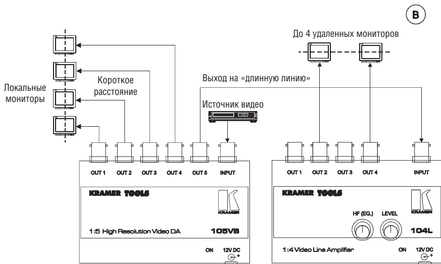
Рис. 11. Линейное усиление сигнала для передачи по длинному кабелю
